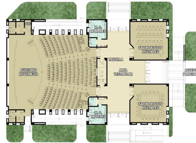
PLANTA ARQUITECTONICA
